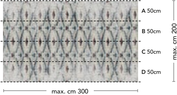
Sviluppo per schienale Decor Panel WDP_122
