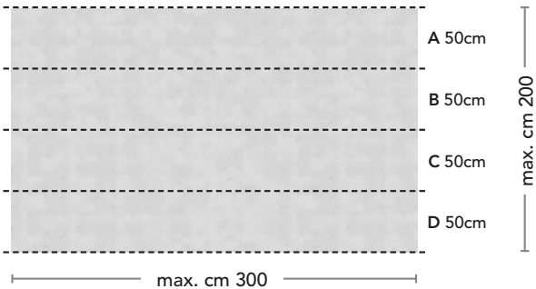
Sviluppo per schienale Decor Panel WDP_810
