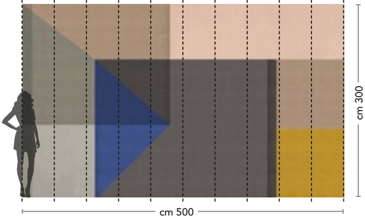
Sviluppo per schienale Decor Panel WDP_844
