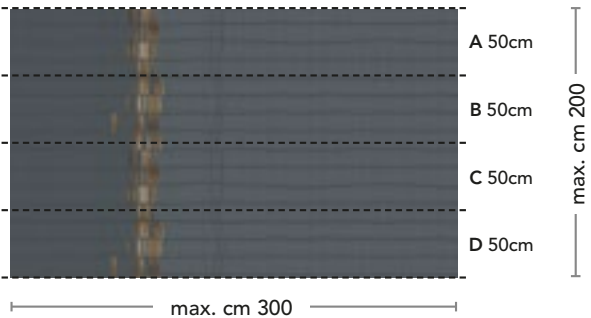
Sviluppo per schienale Decor Panel WDP_854
