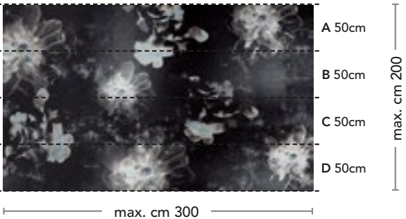
Sviluppo per schienale Decor Panel WDP_622
