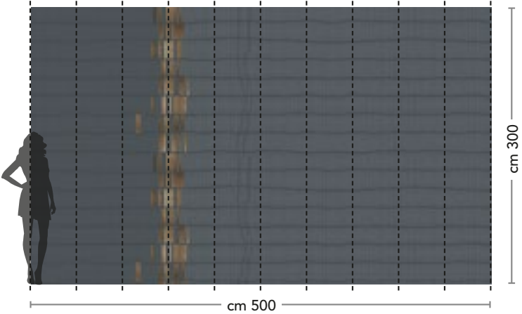
Sviluppo per schienale Decor Panel WDP_854
