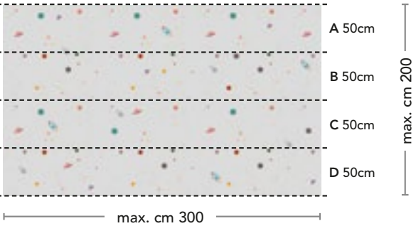
Sviluppo per schienale Decor Panel WDP_723
